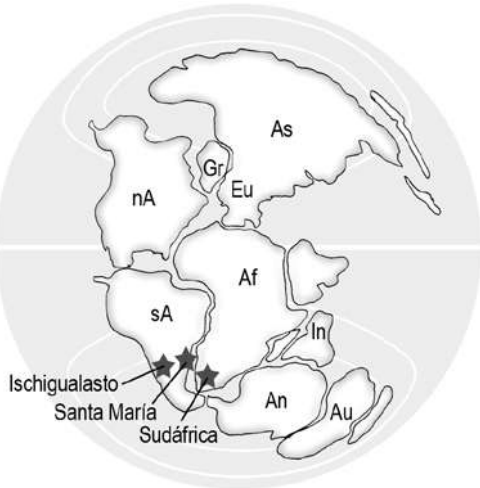
10.13. El sur de Gondwana a inicios del Triásico nos cuenta una de las historias más interesantes del drama de la vida.
