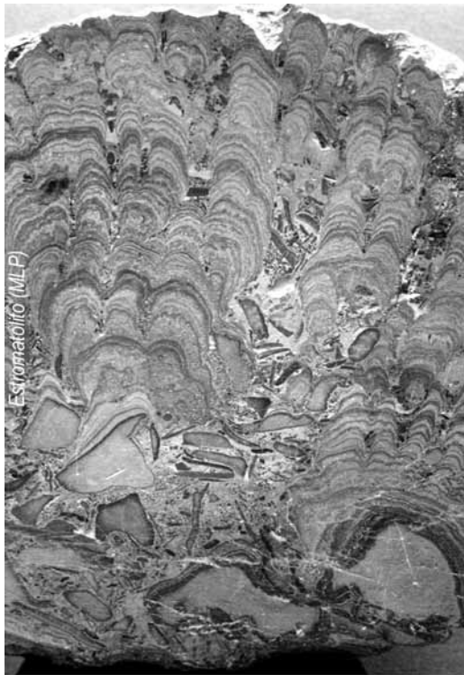
4.4. Corte de una roca que contiene fragmentos de estromatolitos.
