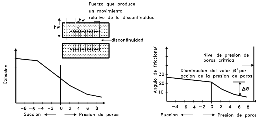
Figura 6.9 Variación de cohesión y el ángulo de fricción dentro de una discontinuidad por el aumento de la humedad y de la presión de poros.
