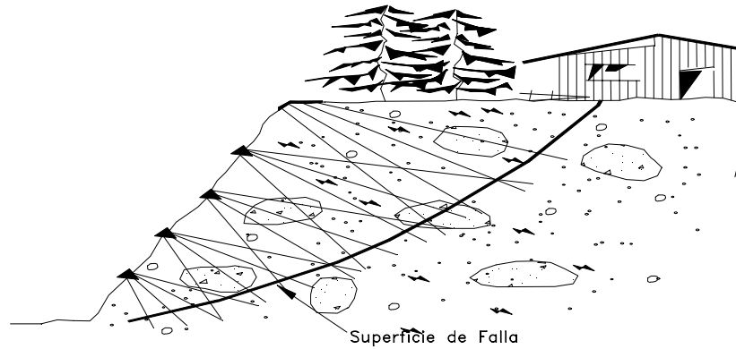
Figura 14.35 Raíces de micropilotes (Root-piles) Lizzi 1977.
