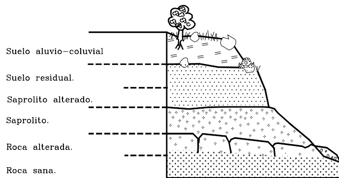
Figura 6.16 Esquema de algunos perfiles típicos en materiales residuales.
