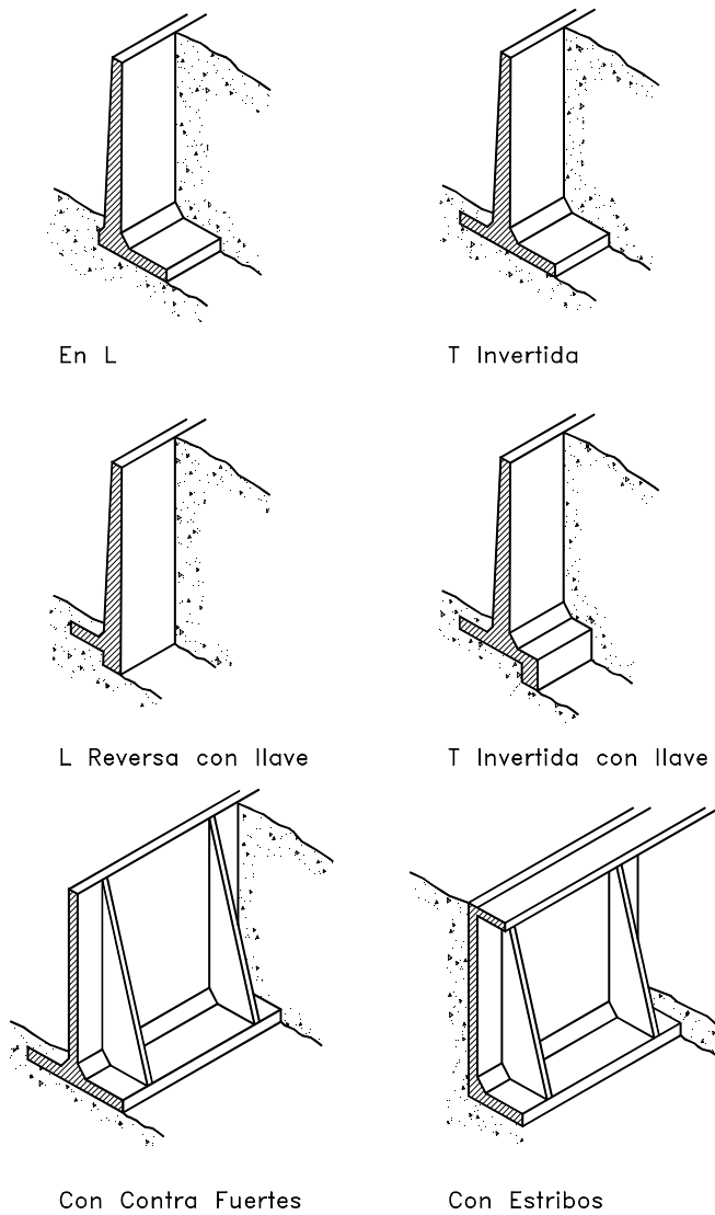
Figura 14.8 Tipos de muro de contención en concreto armado.
