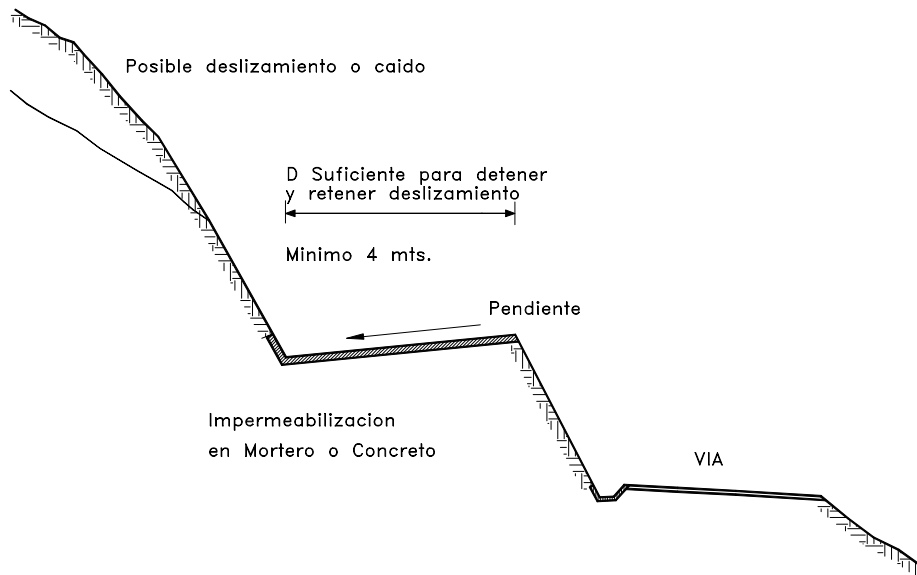
Figura 12.2 Bermas para detener caídos o derrumbes de roca o suelo.
