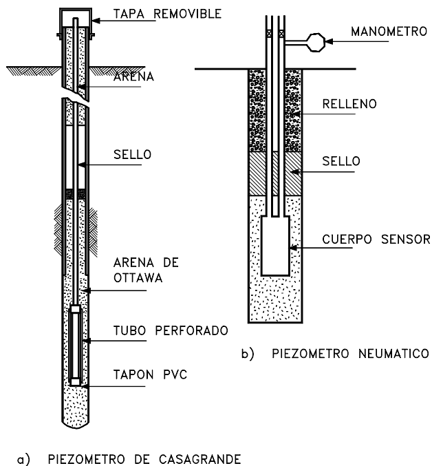
Figura 2.21 Esquema general del piezómetro de Casagrande y piezómetro neumático.
