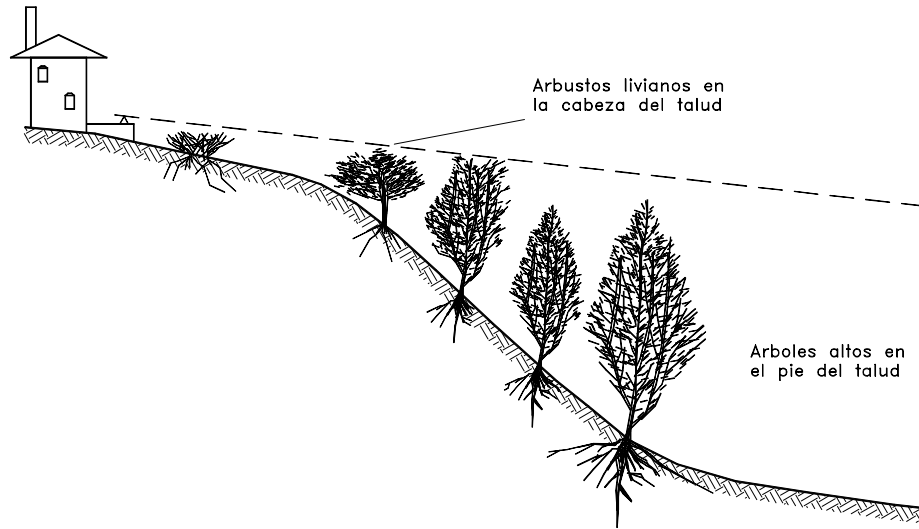
Figura 8.12 Elementos de arquitectura y paisajismo en el diseño de revegetación.
