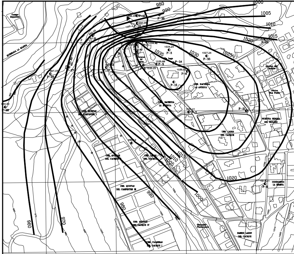
Figura 10.9 Líneas de nivel freático inducidas por la infiltración de un tanque de almacenamiento de agua que produjo el deslizamiento de la Colina en Bucaramanga – Colombia-1996.
