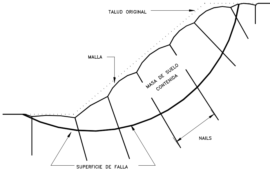
Figura 14.34 Procedimiento de estabilización utilizando "nails" y Malla.
