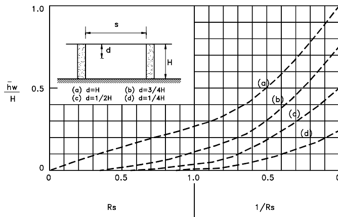
Figura 13.16 Variación de la presión de poros promedio con el espaciamento de subdrenes de zanja (Bromhead, 1984).
