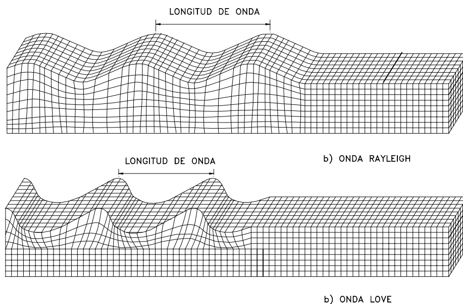
Figura 9.5 Ondas Superficiales.
