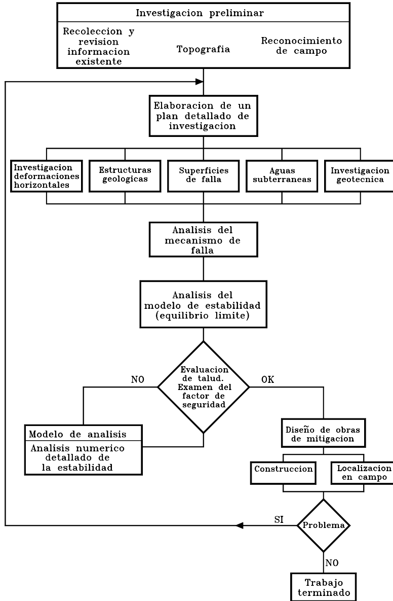
Figura 2.1 Diagrama de flujo para la investigación y análisis de deslizamientos (Japan Landslide Society, 1996).
