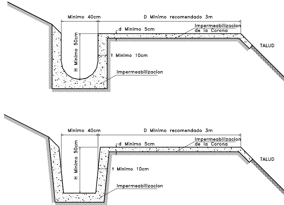
Figura 13.1 Detalle de zanjas de coronación para el control de aguas superficiales en un talud.
